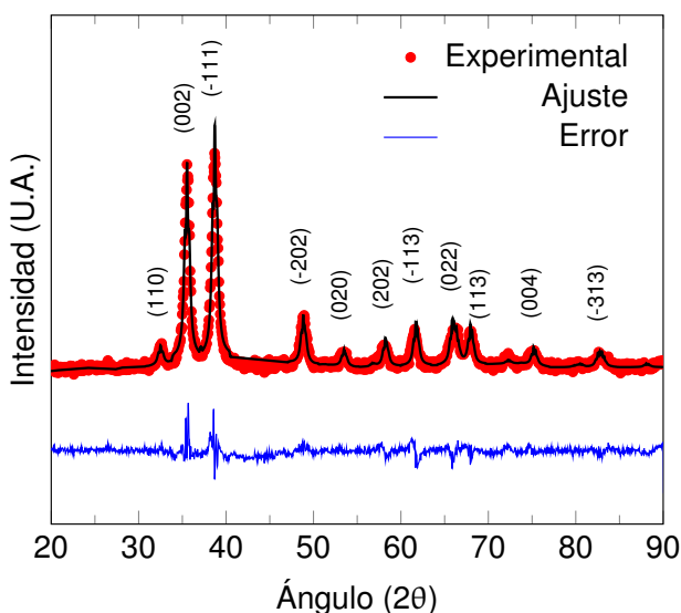
Figura 1: Difractograma de rayos X de NPs CuO; los planos cristalográficos característicos y que coinciden con la carta PDF Card No.: 01-089-5897 Quality: S [3].
